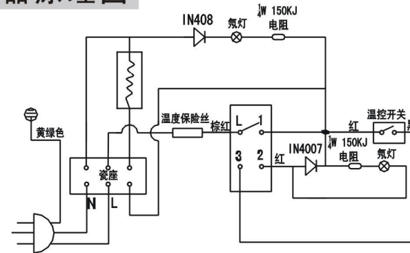
JYZS-M201电器原理图
