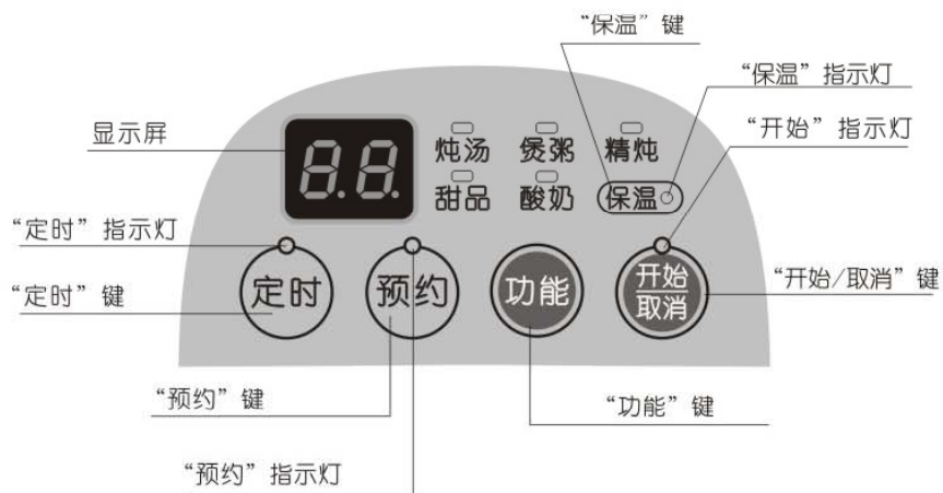
DGW1601AS/DGW1601BS操作面板
