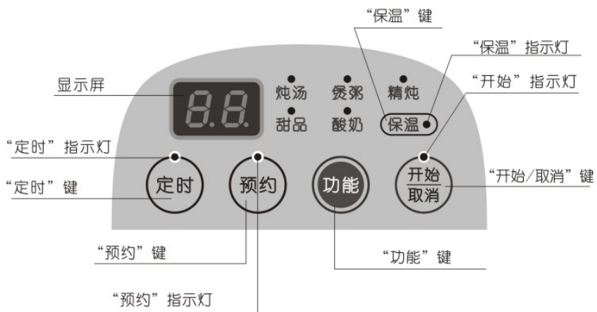
DGW1601AS操作面板
